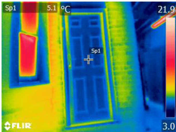
A Citadel Dual Rebate Composite Door
